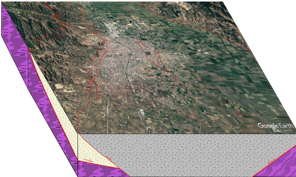
Şekil 5- Aydın'ın genel yeraltı yapısı. Kırmızı çizgiler diri fayları, mor alanlar kaya türü zeminleri noktalı sarı ve gri alanlar eski ve yeni alüvyonları göstermektedir.
