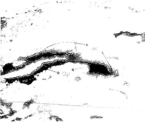
Şekil 8* Opak mineral/Plajioklas dokanakiannında gelişen granat koronaları. Paralel niçoller, 10X. Op= Öpakmin, Gr= Granat Plj= Plajioklas
