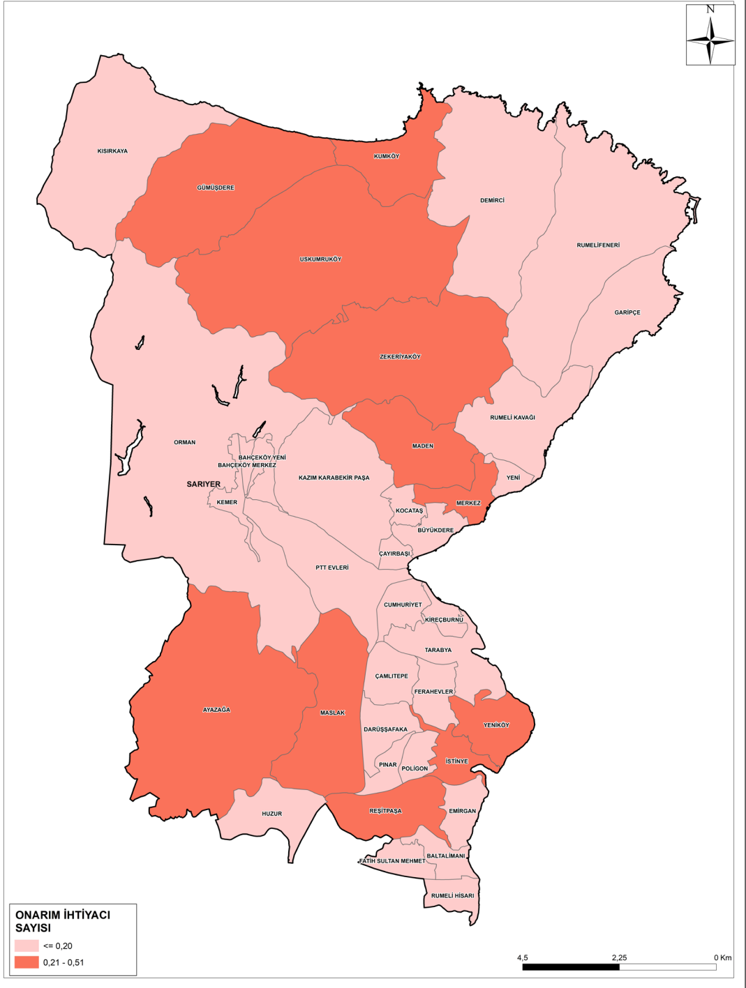
Şekil 5-12: Mw=7.5 Senaryo Depremi İçin Sarıyer İlçesi İSKİ İçme Suyu Boru Hatları Tahmini Onarım İhtiyacı Dağılım Haritası
