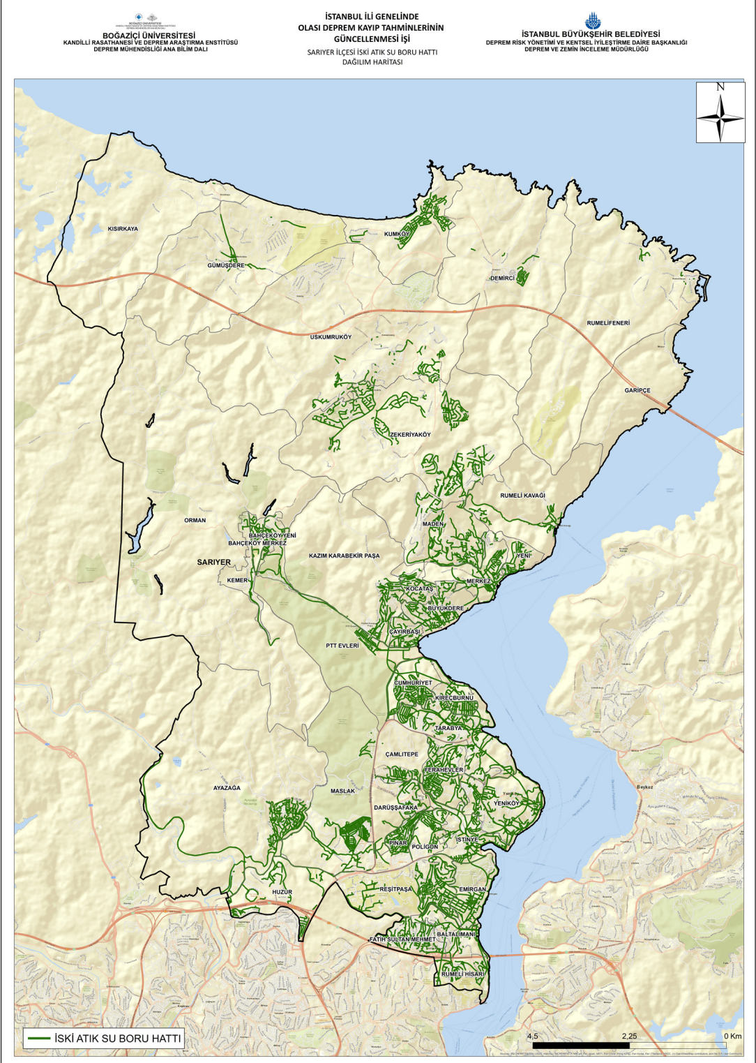
Şekil 3-11: Sarıyer İlçesi İSKİ Atık Su Boru Hattı Dağılımları
