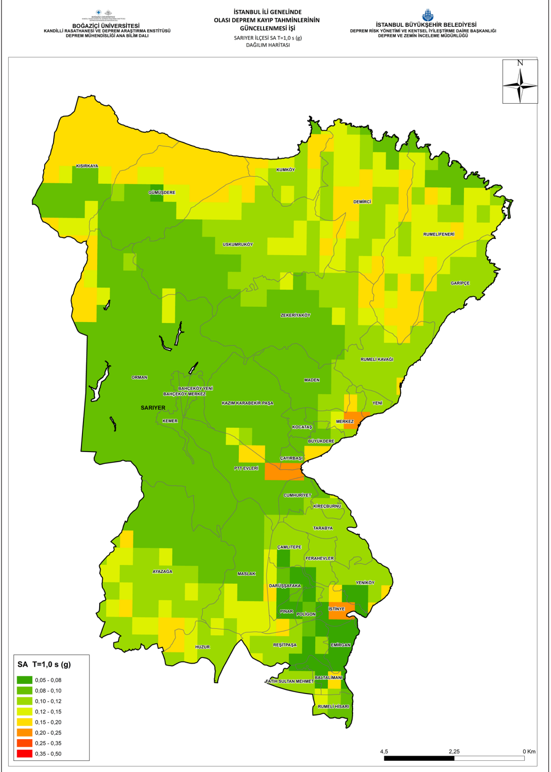
Şekil 4-7: Senaryo Depremi için Elde Edilen Sarıyer İlçesi Zemin Bağımlı T=1.0 s için Spektral İvme Dağılımı
