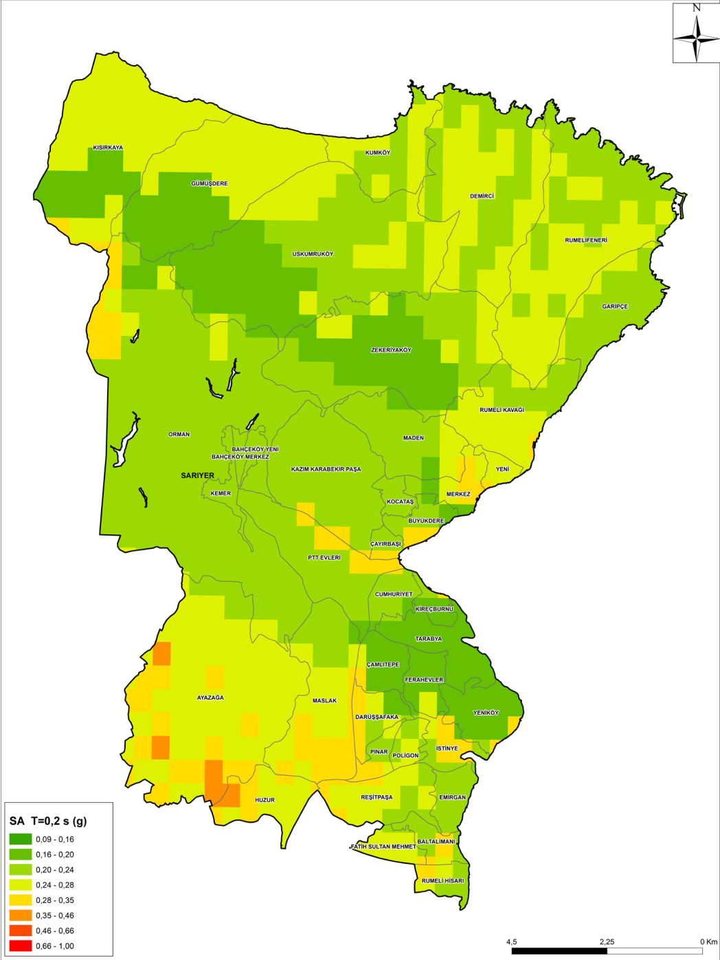
Şekil 4-6: Senaryo Depremi İçin Elde Edilen Sarıyer İlçesi Zemin Bağımlı T=0.2 s İçin Spektral İvme Dağılımı
