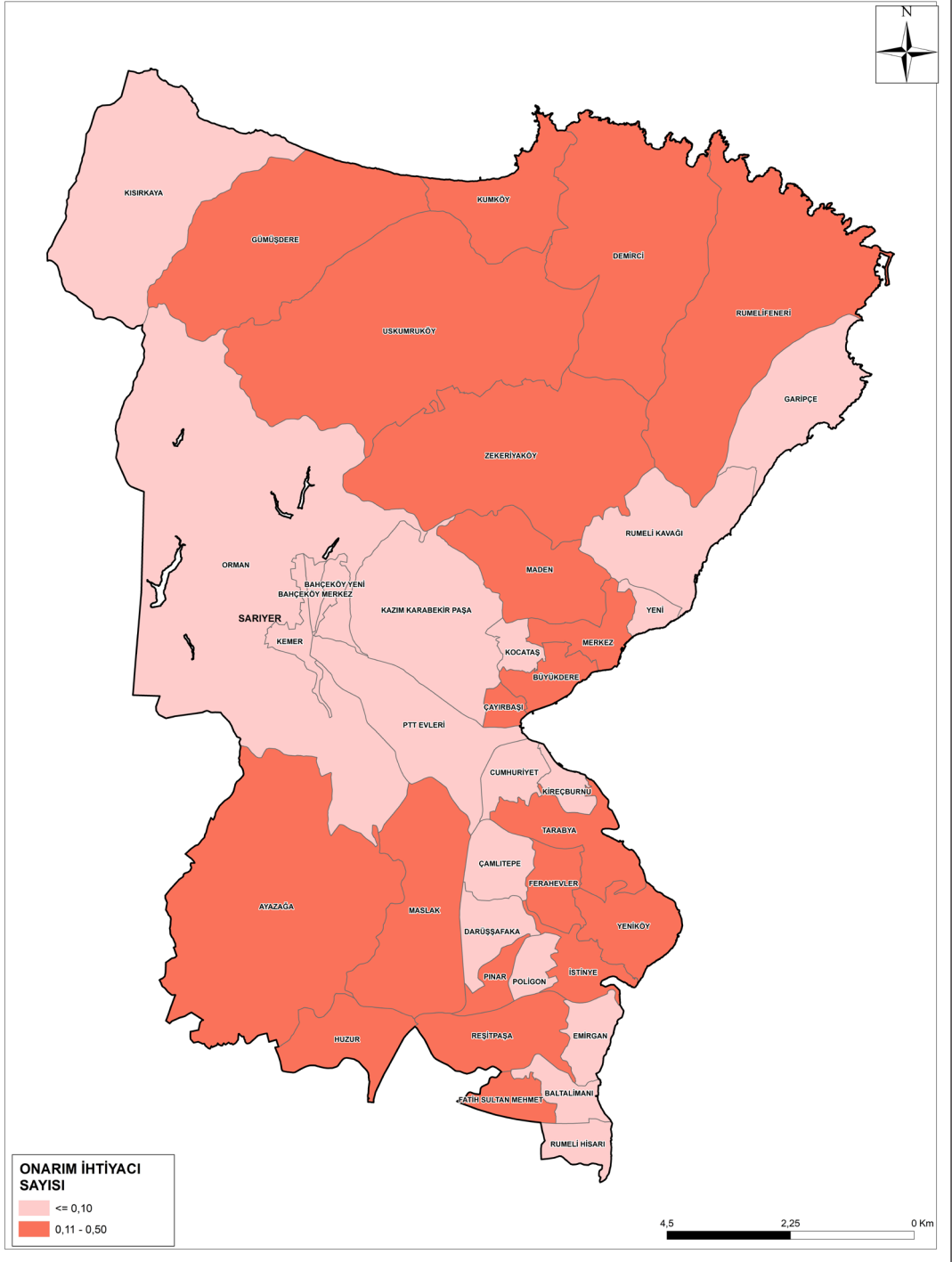
Şekil 5-10: Mw=7.5 Senaryo Depremi İçin Sarıyer İlçesi Doğal Gaz Şebekesi Boru Hatları Tahmini Onarım İhtiyacı Dağılım Haritası
