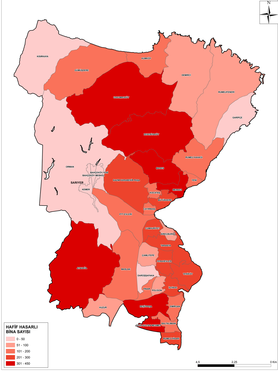
Şekil 5-5: Mw=7.5 Senaryo Depremi İçin Sarıyer İlçesi Tahmini Hafif Hasarlı Bina Sayısı Dağılım Haritası
