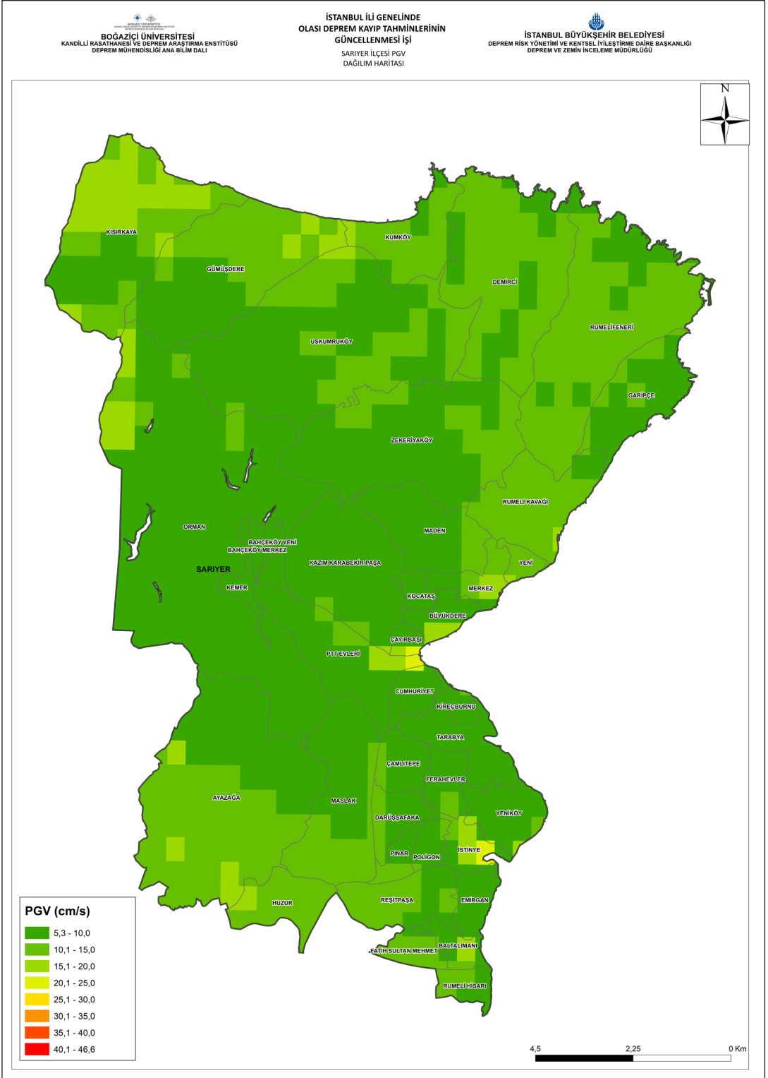
Şekil 4-5: Senaryo Depremi için Elde Edilen Sarıyer İlçesi Zemin Bağımlı Medyan En Büyük Yer Hızı (PGV) Dağılımı
