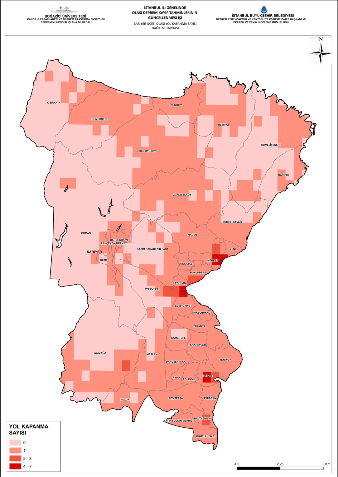
Şekil 5-13: Mw=7.5 Senaryo Depremi İçin Sarıyer İlçesi Yol Kapanma Dağılım Haritası
