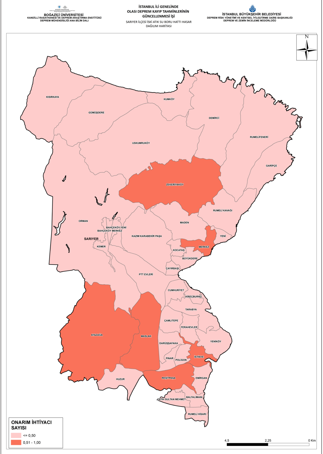
Şekil 5-11: Mw=7.5 Senaryo Depremi için Sarıyer İlçesi İSKİ Atık Su Boru Hatları Tahmini Onarım İhtiyacı Dağılım Haritası
