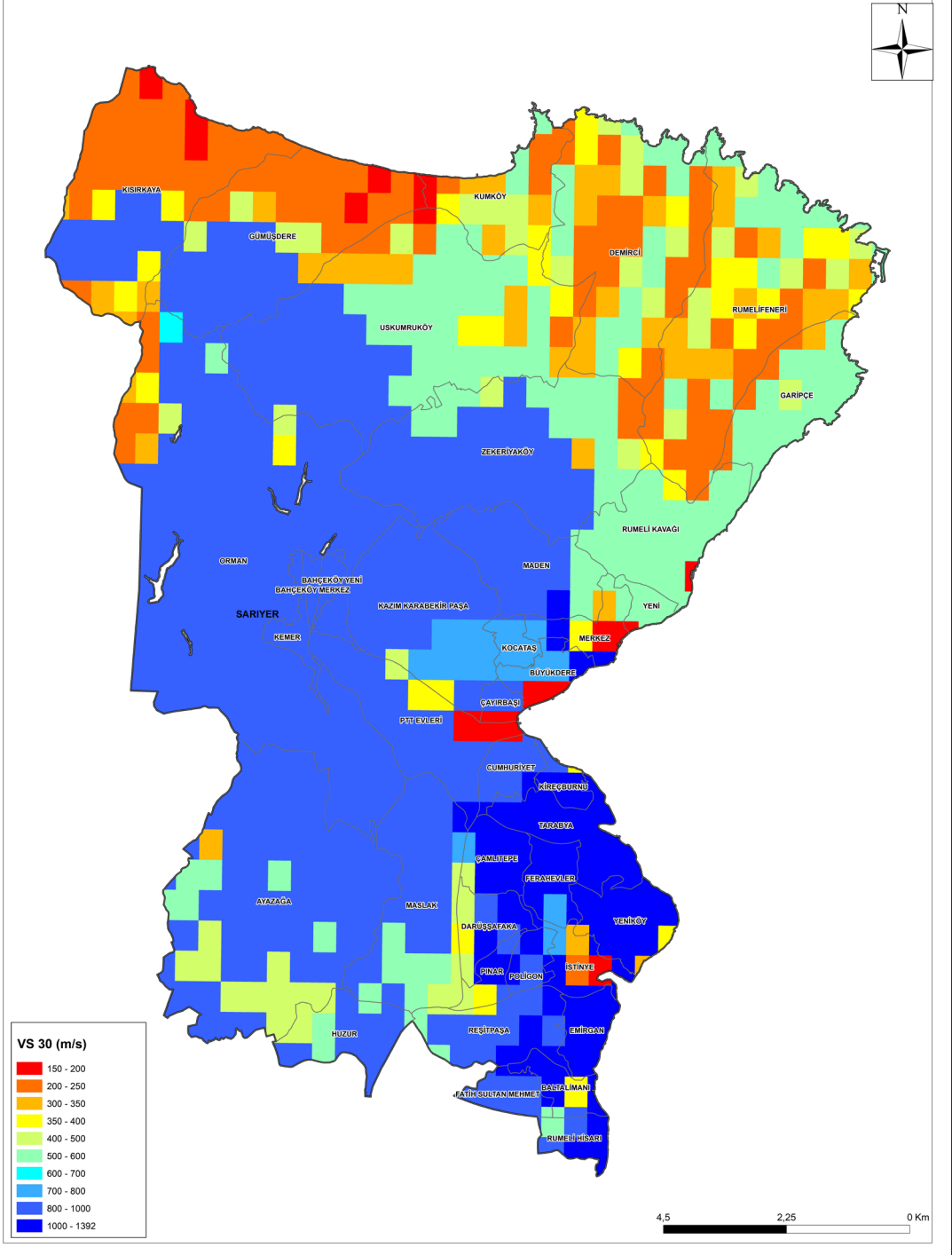
Şekil 4-1: Sarıyer İlçesi VS 30 Dağılımı
