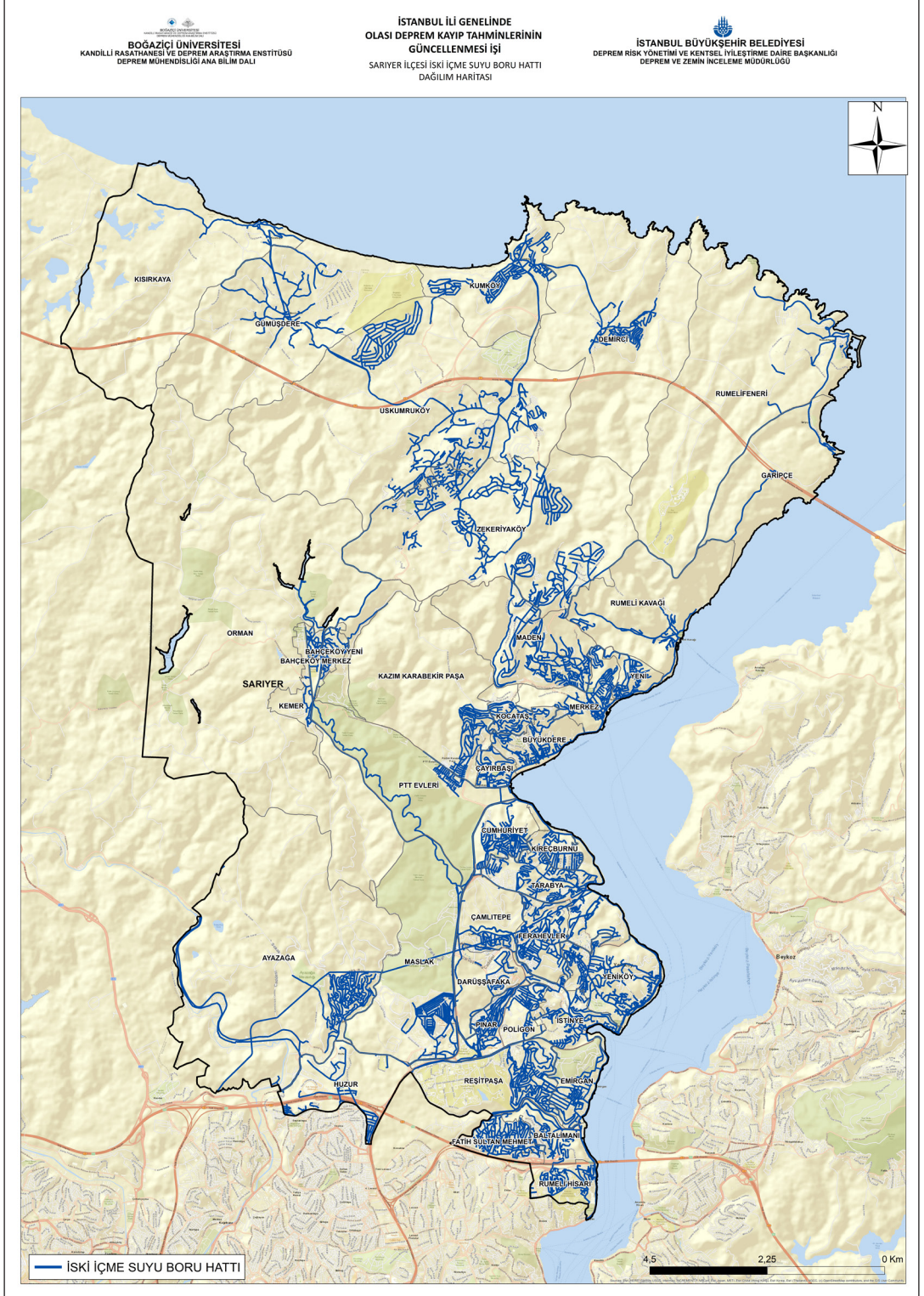
Şekil 3-10: Sarıyer İlçesi İSKİ İçme Suyu Boru Hattı Dağılımları
