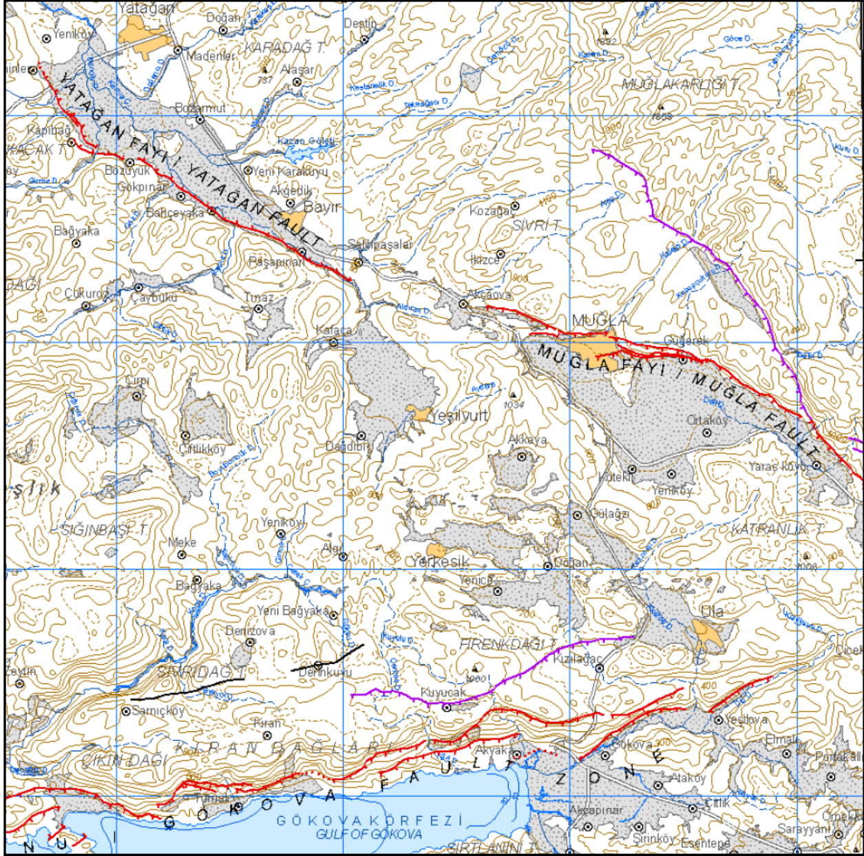
Şekil 3- TDFH'na göre Muğla ve çevresindeki diri faylar (Duman vd., 2011). Kırmızı ve mor renkli kalın çizgiler diri faylar, siyah çizgiler ise olası diri faylardır. Gri renkli alanlar alüvyon çökellerini gösterir.
