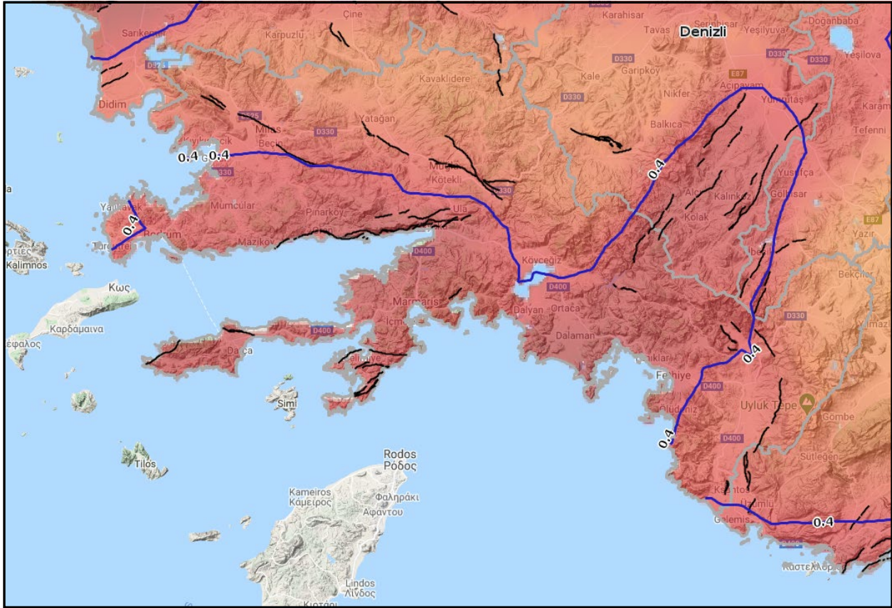
Şekil 1- Muğla ili Deprem Tehlike Haritası ( https://tdth.afad.gov.tr/TDTH/main.xhtml ).
