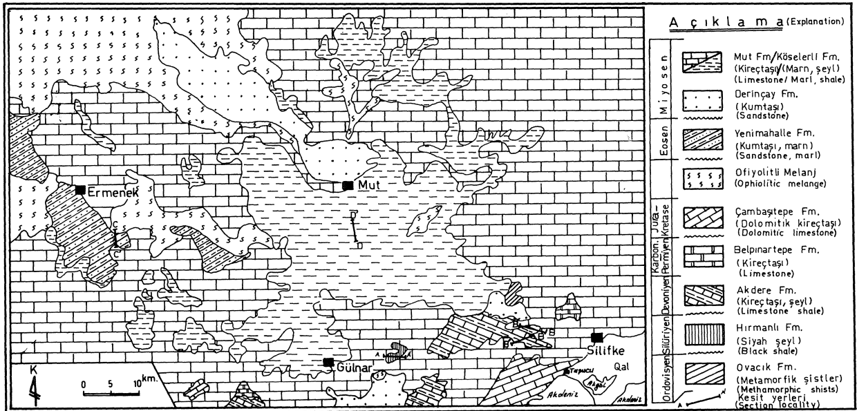
Şekil 2: Mut-Ermenek-Silifke havzasının sadeleştirilmiş jeolojik haritası (Gedik ve diğ., 1979'dan)
