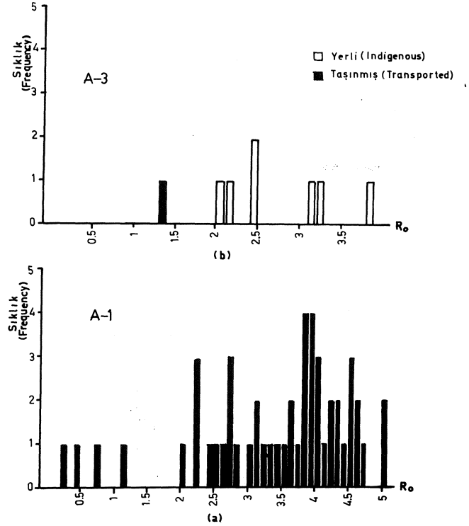
Şekil 6: Devoniyen yaşlı Akdere Formasyonu'na ait örneklerdeki vitrinit dağılımları.
