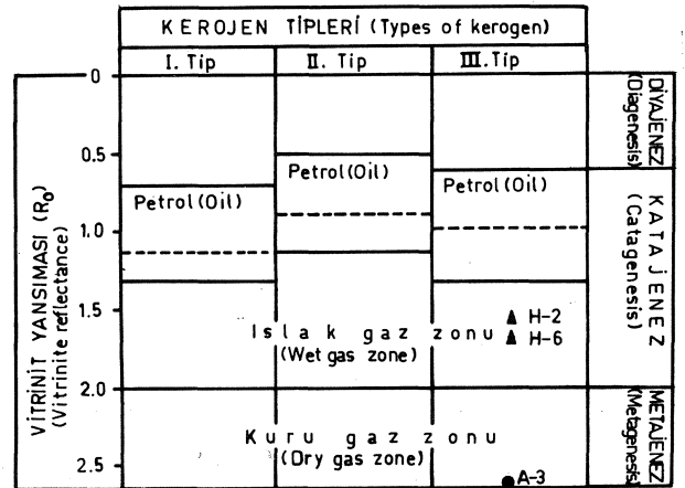
İk Hırmanlı Form. (Silüriyen) # Akdere Form. (Devoniyen)
