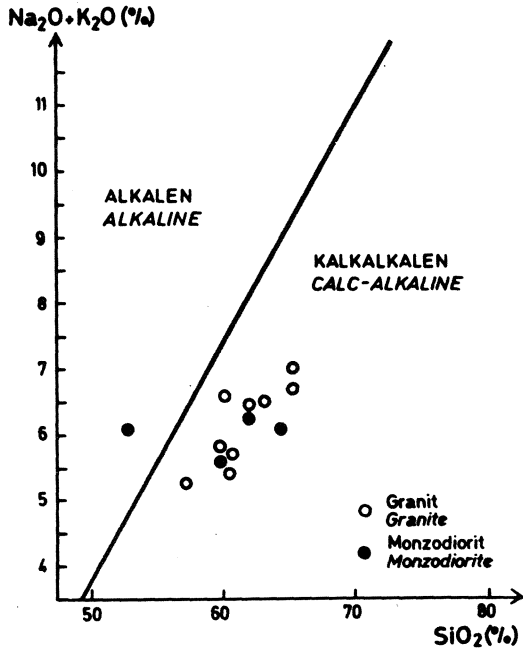
řekil 17. Beypazarı granitinin (Na_2O+K_2O)/SiO_2 diyagramı.
