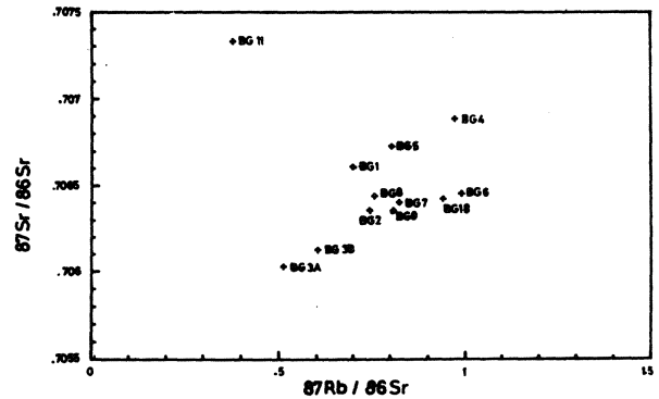
řekil 19. ^{87}Sr/^{86}Sr izotop oranı analiz sonuçları.
