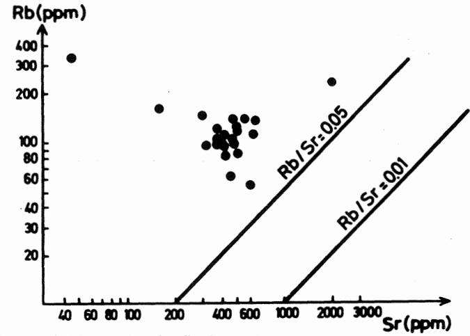
Şekil 16. Granite Rb/Sr oranları.
