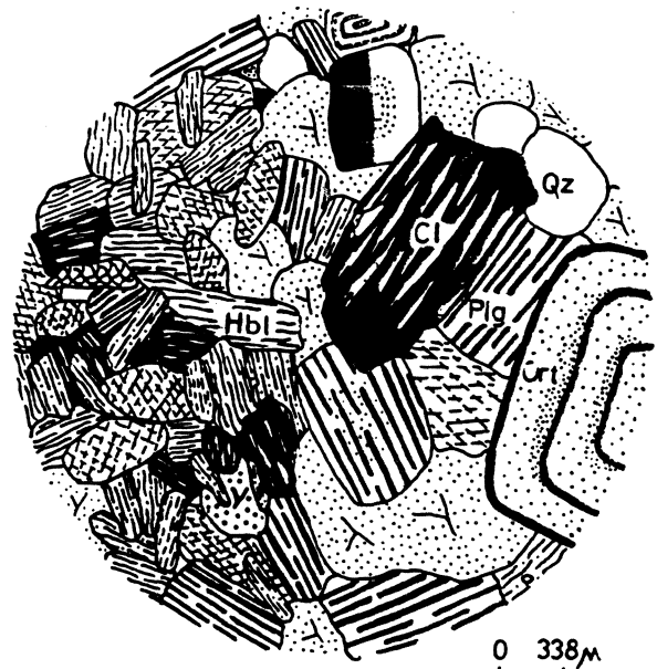
Şekil 9. Granit ile anklavın kesin sınırı.
