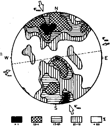
ekil 13: Mermerlerde do rultuda alınan ince kesitlerin U tabanlı mikroskopta incelenmesi ile bulunan optik eksen (C) do rultularına göre hazırlanan yönelim diyagramı.
