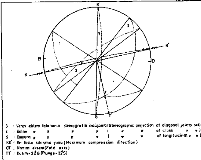
ekil 8B: Eklem takımlarının ve antiklinalin stereografik izdüşümü. Figure 8B: Stereographic projection of joints sets and anticlinal.
