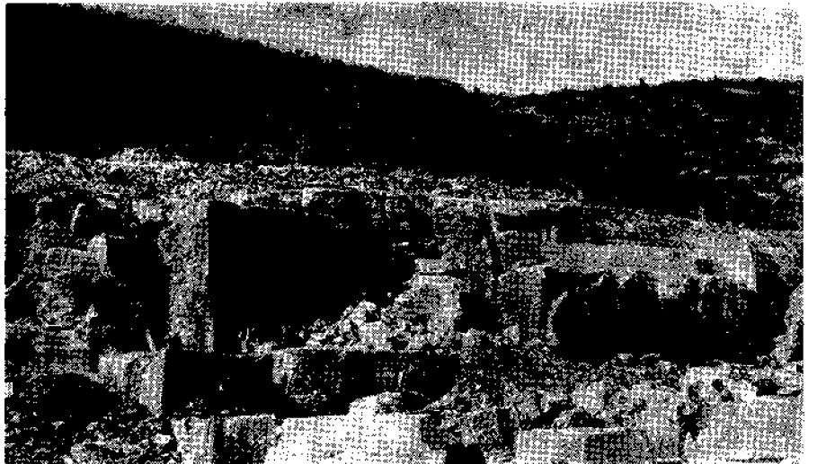
Şekil 3: Marmara Adasındaki mermer ocağında DB ve KG doğrultusunda belirgin olarak görülen gerilme çatlakları. Figure 3: Apparent tension cracks in EW and NS directions, in a marble quarry, in Marmara Island.
