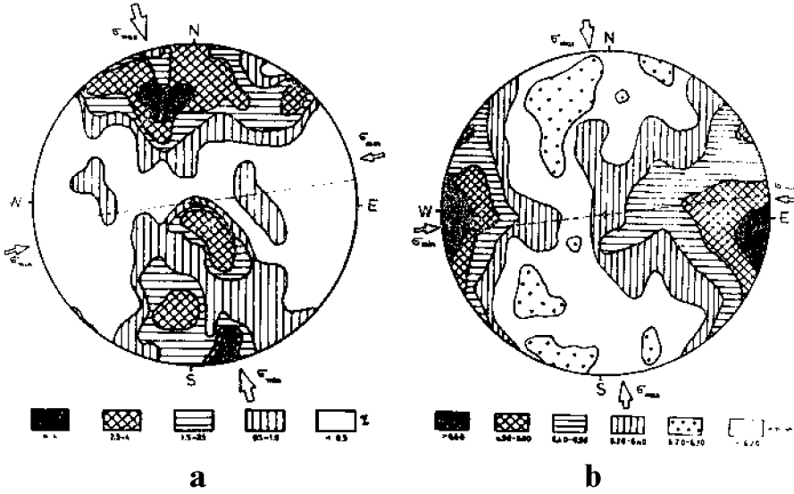
Şekil 14: Optik eksen yönelim diyagramı (a) ve elastik anizotropi (b) diyagramlarındaki bakımlılığa göre saptanan gerilme ( \sigma_1 ve \sigma_2 ) doğrultuları.
