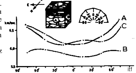
Şekil 10: Foliasyona dik ve paralel do rultuda hazırlanan üç 12 gen örnekte ölçölen hız de erleri göre hazırlanan hız da ılımı diyagramı.
