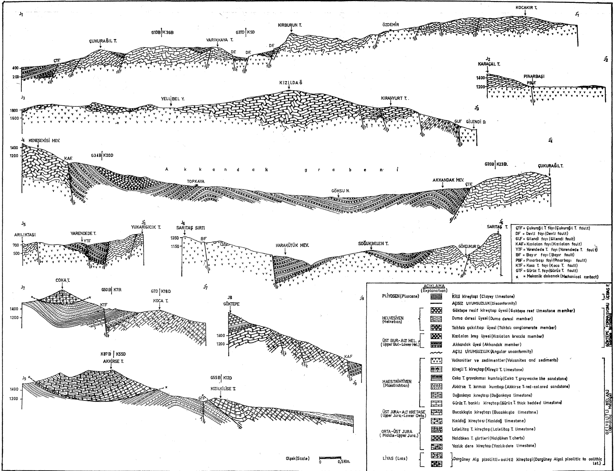
Sekil 6: Karaman-Ermek (Konya) arasındaki bölgenin jeolojik kesitleri. Figure 6: Geologic cross-section of the region between Karaman-Ermek (Konya).
