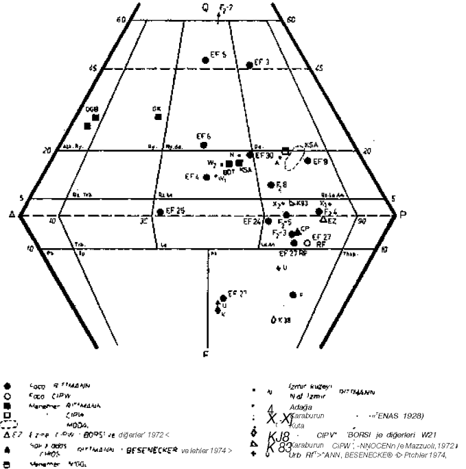
Şekil 2: Foça, Menemen ve öteki bazı Batı Anadolu volkanitlerinden örnek kayaların, çe itli normlara göre Streckeisen çiftüçgenindeki yerlemi. Figure 2: The representative specimens from Foça, Menemen and other localities of W Anatolia, calculated to different norms plotted in Streckeisen's doubletriangle.
