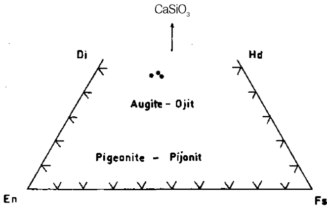
Şekil 6: Gümüşhane piroksen-andezitlerindeki ojit'in bileşimi (Analiz elektron prob'da yapılmıştır).
