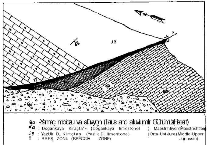
ekil 7: Manastır D. mekanik dokanağını gösterenematik profil. Figure 7: The schematic profile showing Manastır D. mechanical contact.
