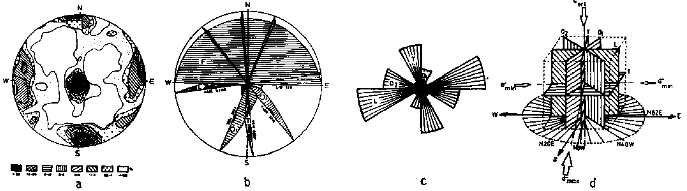
Şekil 4: a) Mermerlerde ölçülen çatlaklarla hazırlanan kontur diyagramı. b) Kontur diyagramındaki egemen doğrultuları temsil eden çatlakların stereografik izdüm diyagramı. c) Arazide ölçülen çatlakların türümsel sınıflandırılması. L: Boyuna çatlak (Gerilme çatlak) T: Enine çatlak (Gerilme çatlak) O 1 , O 2 : Oblik çatlaklar (Kesme çatlakları) d) Çatlaklarınematik blok diyagramı ve bunları doğuran gerilme sistemi Q 1 : N 8 W o 1 • K 82 13 min*
