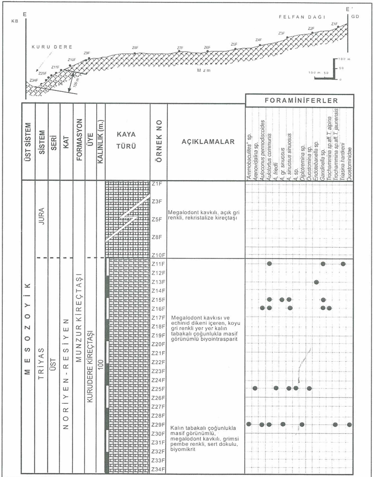
Şekil 5. Kurudere ölçütlü stratigrafi kesiti
