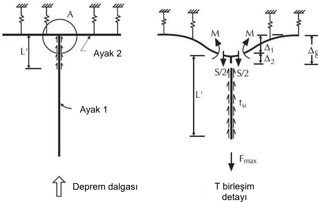
Şekil 5.5. T tipi birleşim noktasında kuvvet ve yerdeğıştirmeler
