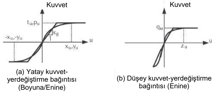
Şekil 7.1 Boru-zemin arayüzü için geçerli olan idealize elastoplastik kuvvet-yerdeğiştirme bağıntıları (O'Rourke, 2012 çalışmasından değiştirilerek alınmıştır)
