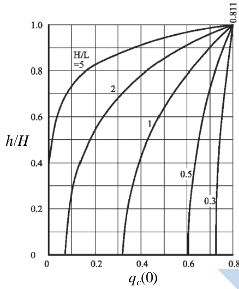
Şekil 4.6 Dikdörtgen kesitli tanklar için devinimsel hidrodinamik basınç katsayısının: (a) yükseklik boyunca değişimi ve (b) katsayının tabandaki değeri
