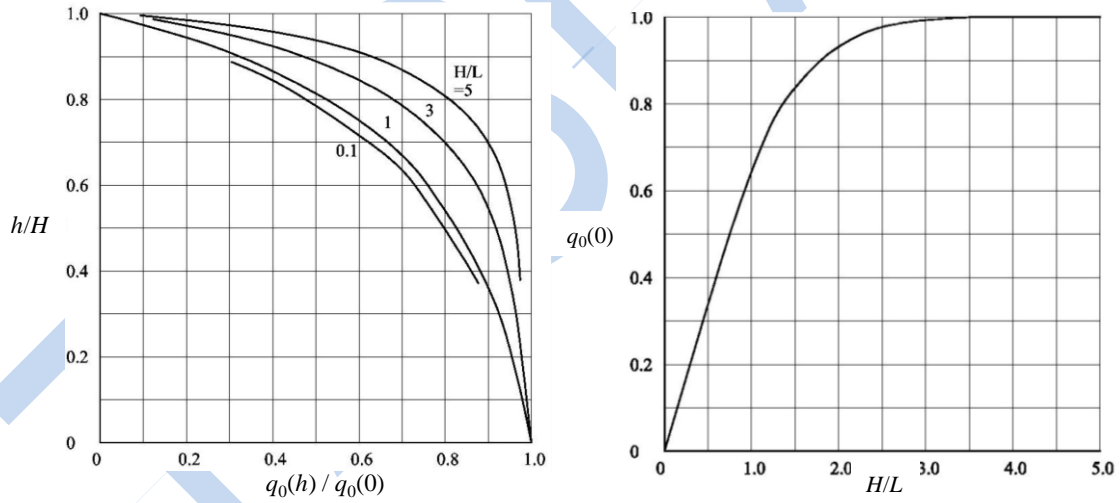
Şekil 4.5 Dikdörtgen kesitli tanklar için darbesel hidrodinamik basınç katsayısının: (a) yükseklik boyunca değişimi ve (b) katsayının tabandaki değeri
