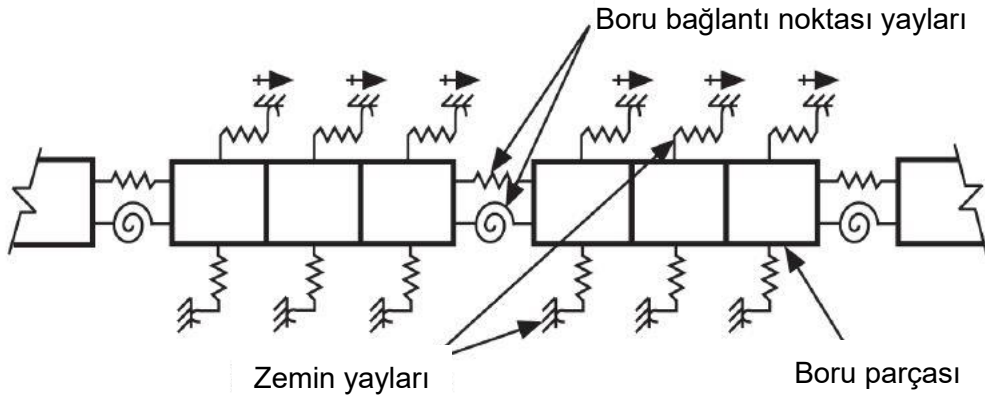
Şekil 7.2. Parçalı boru hattı deprem davranışının belirlenmesinde kullanılabilecek boru-zemin modeli (Wang 1979 çalışmasından değiştirilerek alınmıştır).
