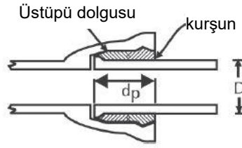
Şekil 8.1. Parçalı boru hattı birleşim noktası birleşim derinliği ( d_p ) temsili resmi
