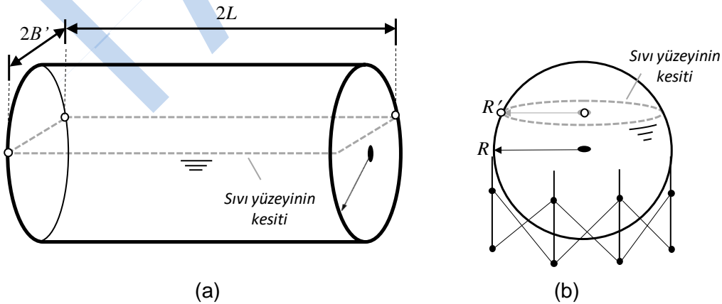
Şekil 4.7 Tank geometrilerinin tanımı: (a) yatay silindirik ve (b) küresel
