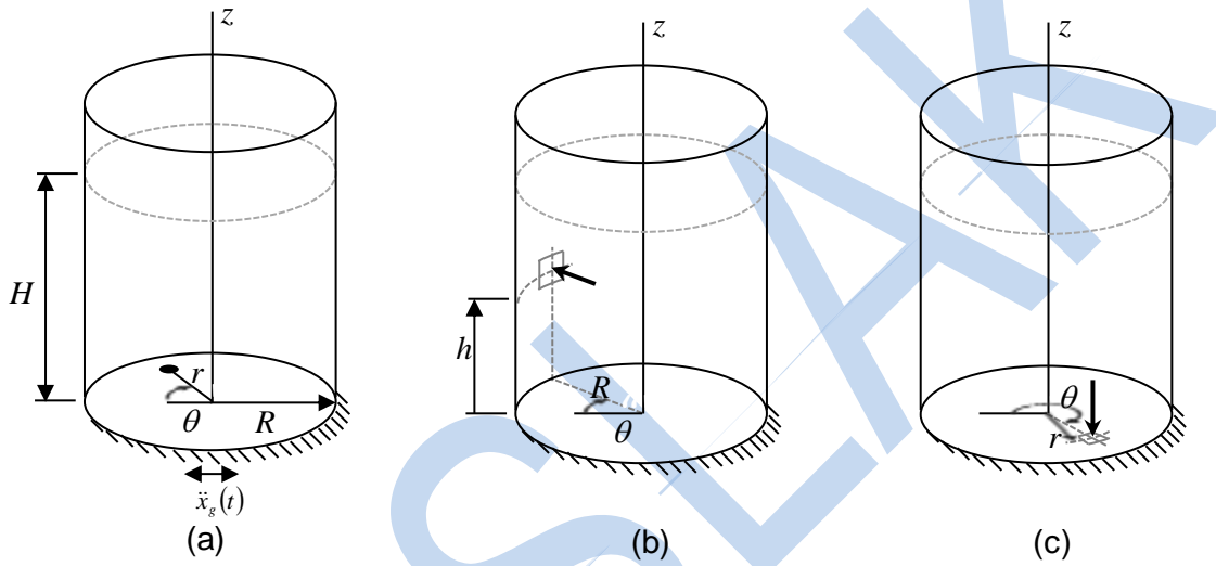
Şekil 4.3 Silindirik tankların analizi için tanımlanan: (a) koordinat sistemi, (b) duvar üzerindeki belirli bir noktaya etkiyen basınç ve (c) tabanda belirli bir noktaya etkiyen basınç.
