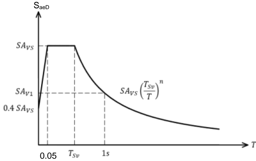
Şekil 2.3. Temsili düşey ivme tasarım spektrumu
