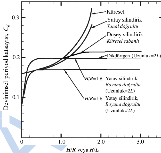
Şekil 4.2 Devinimsel titreşim mode hesaplama katsayısı, C_d (düşey silindirik tanklar haricindeki tank geometrileri için)
