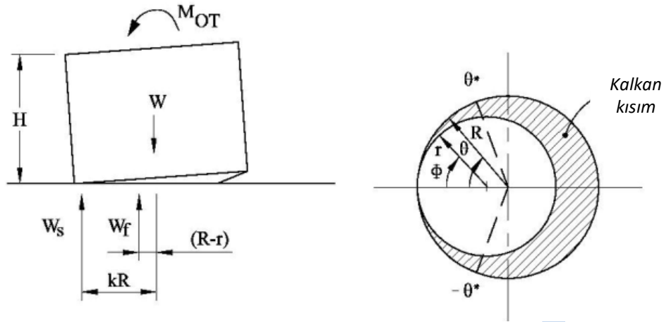
Şekil 4.8 Devrilme momenti etkisi altında tabanın zeminden kalkması (NZS, 2009'dan değiştirilerek alınmıştır).
