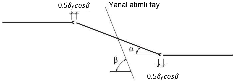
Şekil 6.2 Parçalı boru hattının sağ atımlı bir fayı kesmesi durumu
