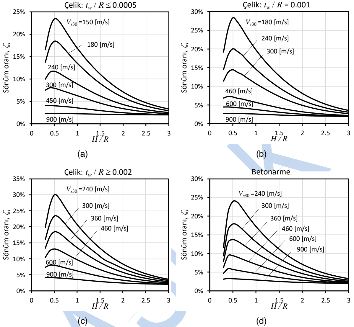
Şekil A.2 Zemin-yapı etkileşimli tanklarda darbesel titreşim modu sönüm oranı, \zeta_i
