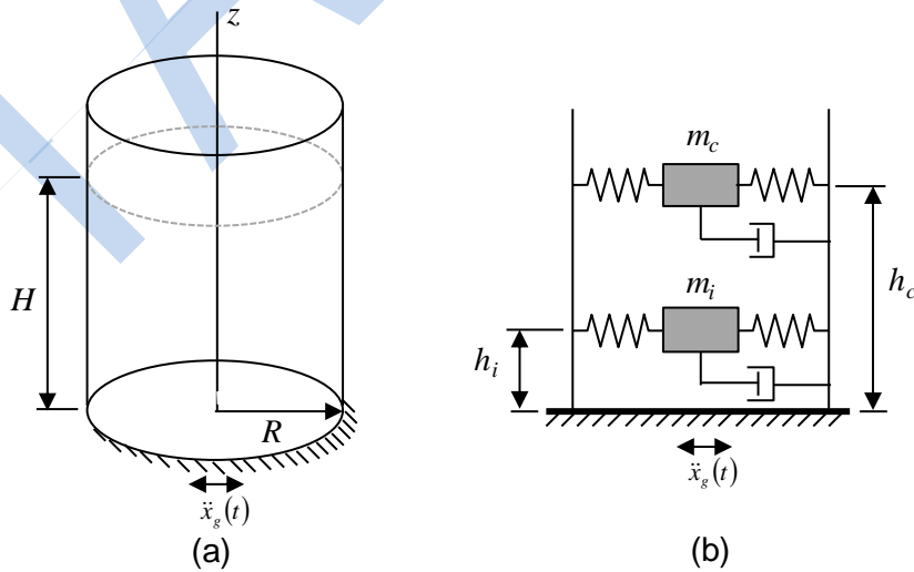
Şekil 4.1 Silindirik tanklar için hesap yüklerinin tanımlanmasında kullanılan: (a) geometri parametreleri ve (b) eşdeğer yığılı kütleli modelleme yaklaşımı.
