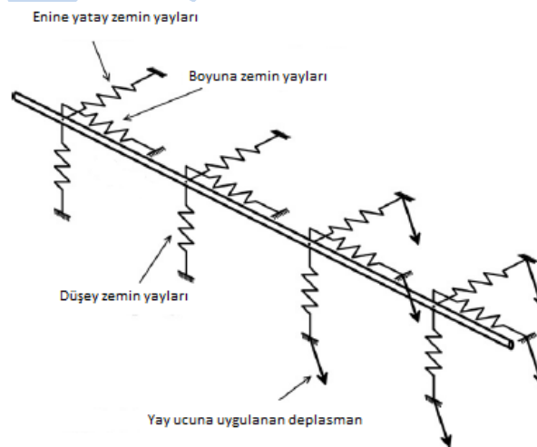
Şekil 7.1. Boru hattı deprem davranışının belirlenmesinde kullanılacak boru-zemin modeli (Karamitros vd. 2011 çalışmasından değiştirilerek alınmıştır).
