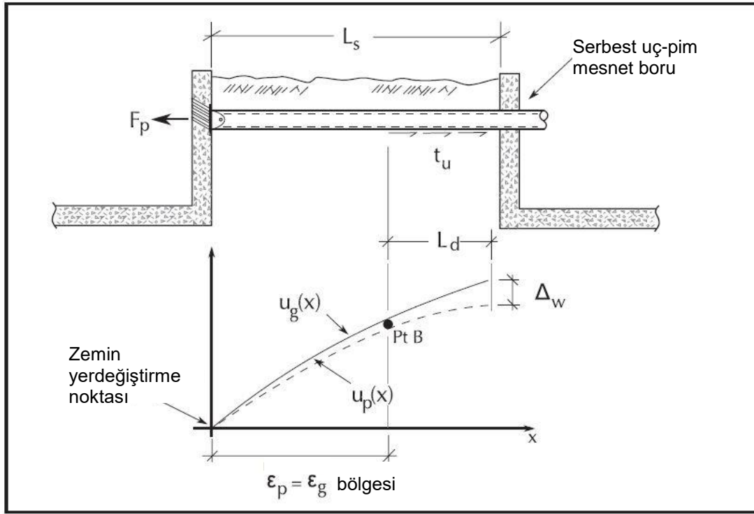
Şekil 5.3 L_s > L_d durumu. O'Rourke ve Liu (2012)'den değiştirilerek alınmıştır.
