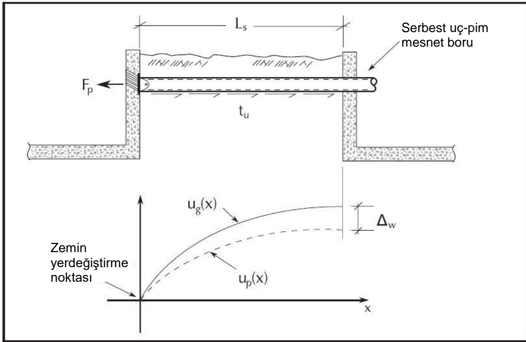
Şekil 5.2 L_d > L_s durumu. O'Rourke ve Liu (2012)'den değiştirilerek alınmıştır.
