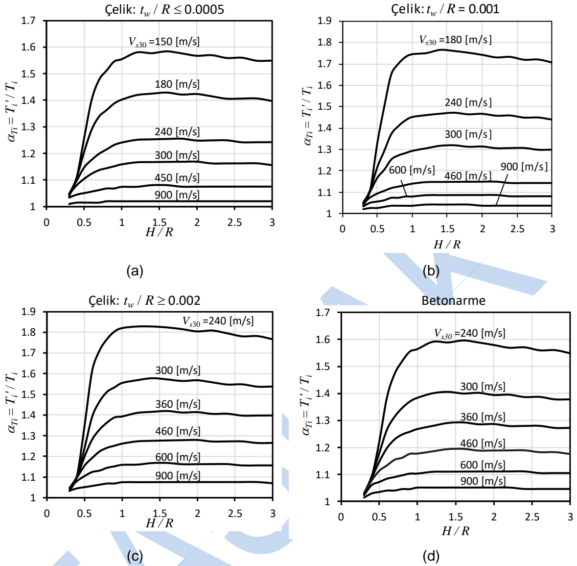
Şekil A.1 Zemin-yapı etkileşimli tanklarda etkili darbesel periyod, T_i' hesaplama katsayısı
