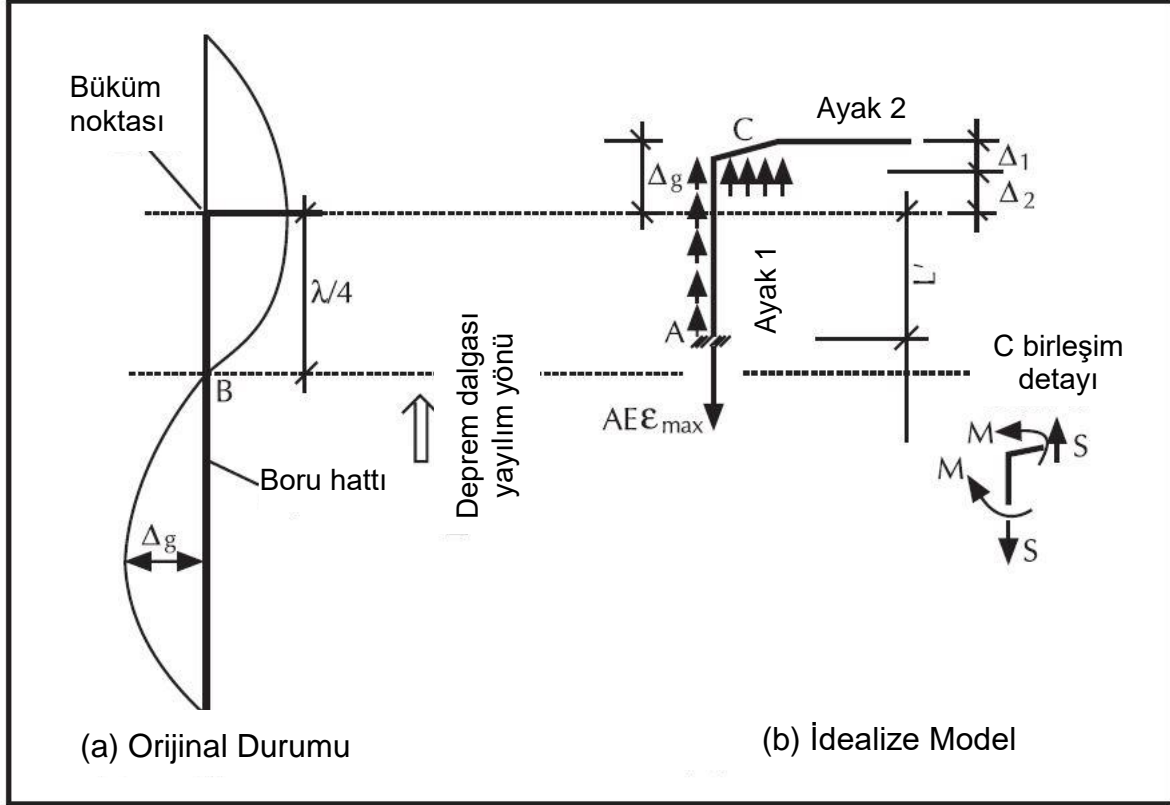
Şekil 5.4 Dirsekli bir boruda yerdeğıştirmeler ve kuvvetler
