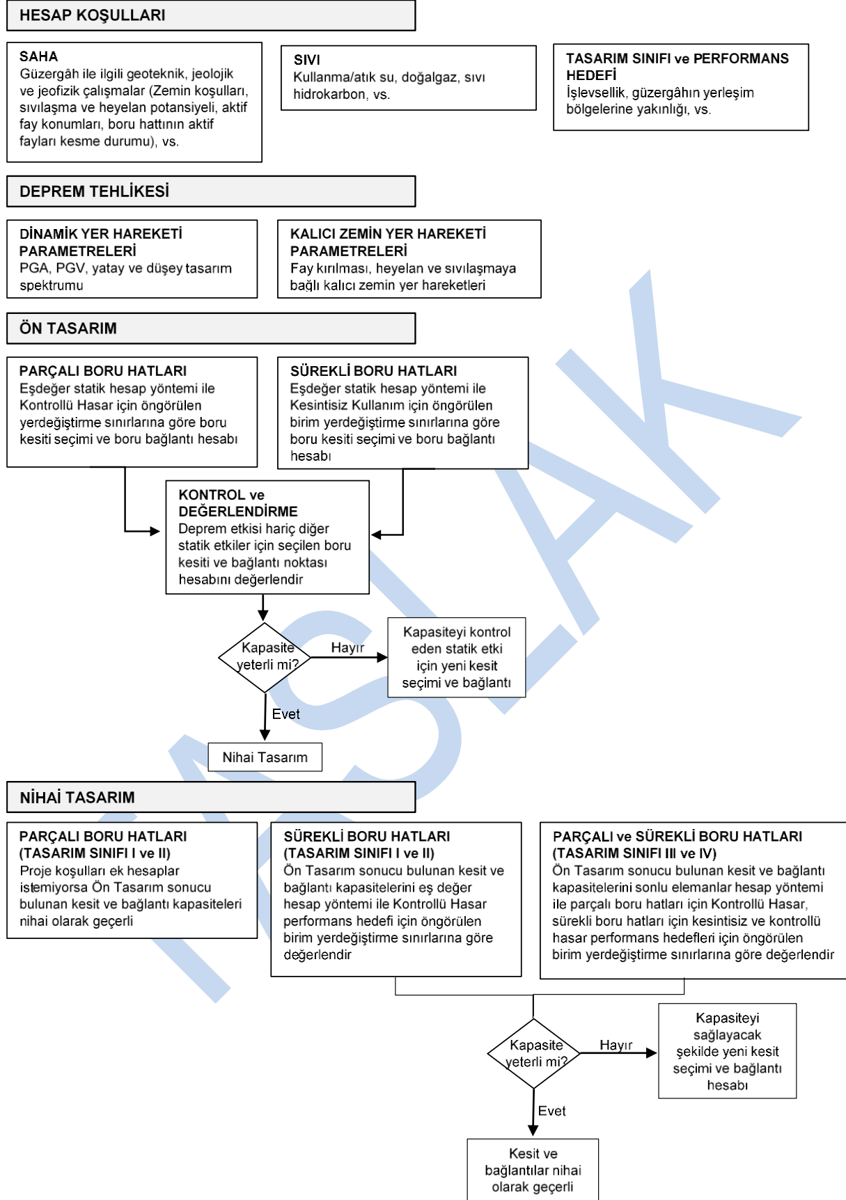
Şekil 4.1. Performans Esaslı Boru Hatları Analiz ve Tasarım Felsefesi
