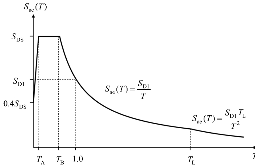
Şekil 2.1. Temsili yatay ivme tasarım spektrumu
