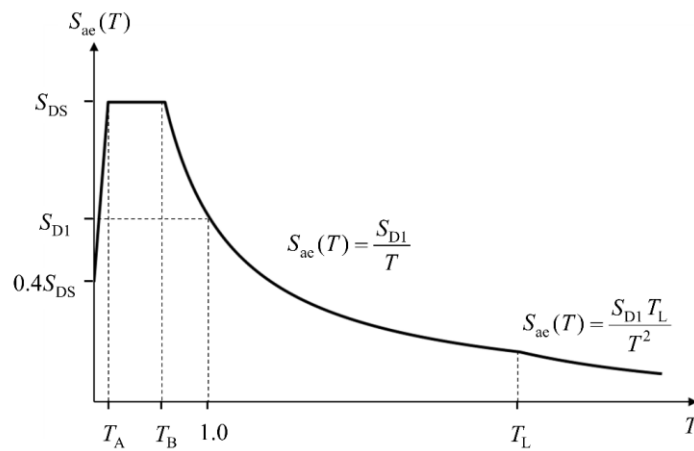
Şekil 2.1. Temsili yatay ivme tasarım spektrumu
