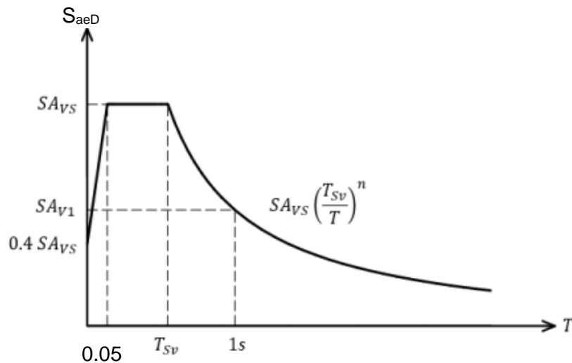
Şekil 2.2. Temsili düşey ivme tasarım spektrumu
