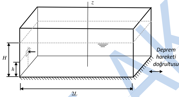
Şekil 4.4 Dikdörtgen sıvı depolama tankı geometrisi
