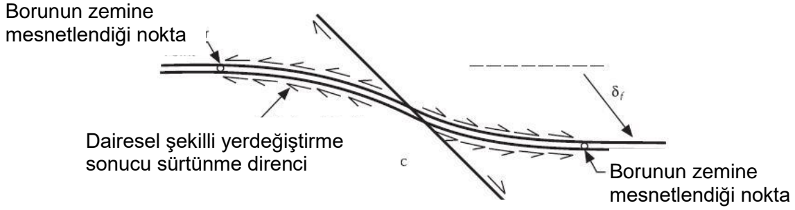
(b) Fay hareketi sonrası
