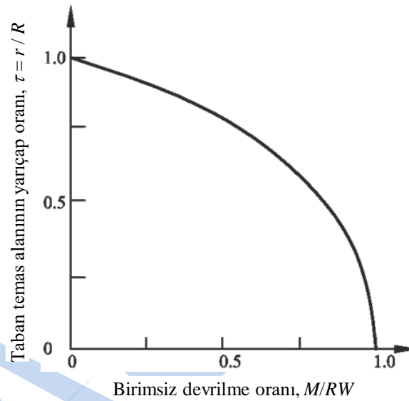
Şekil 4.9 Taban temas alanı yarıçap oranı
