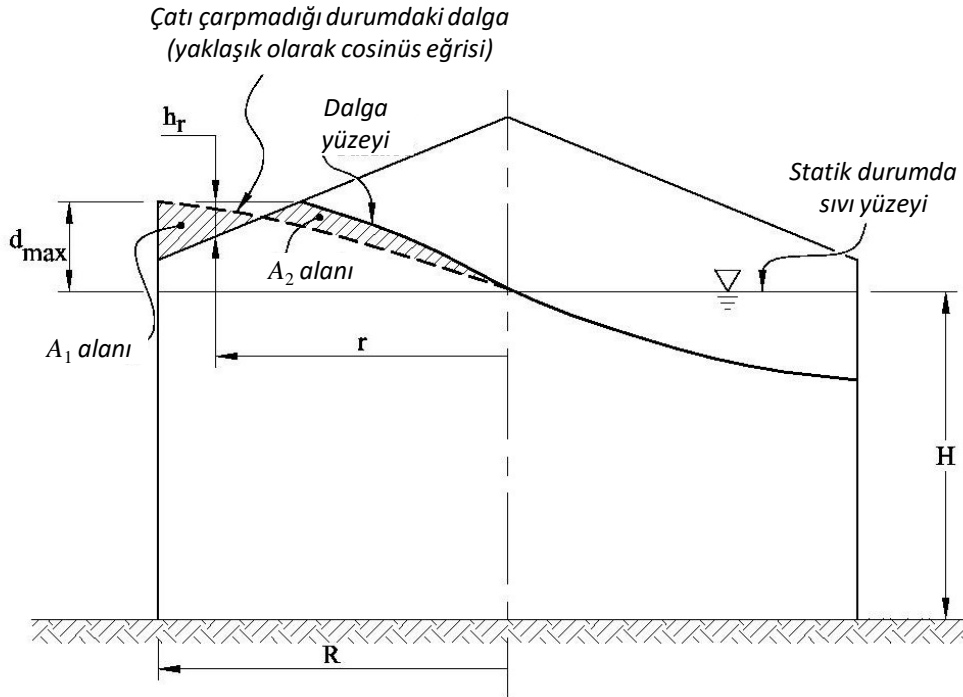
Şekil 4.12 Tank tavanına dalga çarpma etkisinin hesabı
