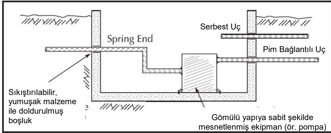
Şekil 5.1. Sürekli boruların gömülü yapılarla bağlantılarında farklı sınır koşulları. O'Rourke ve Liu (2012)'den alıntıdır.
