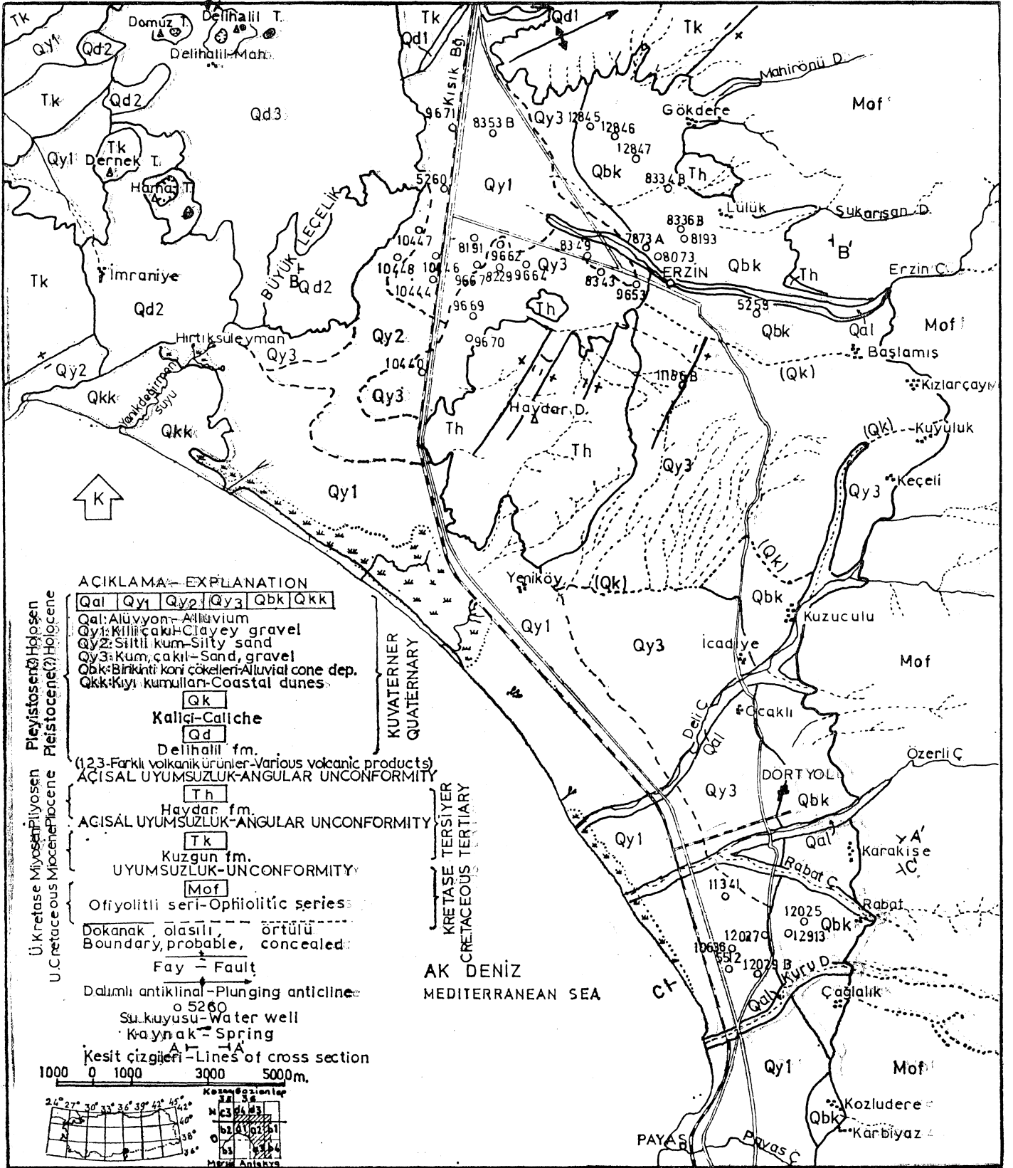
Şekil 4 : Erzin ve Dört Yol ovalarının jeolojik haritası
